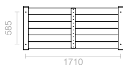
Sicht von darunter (mit Befestigungsmittenabstand)
