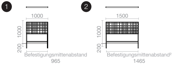
Befestigungsprinzip
