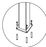
Bodenplatte
