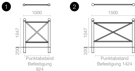
Befestigungsprinzip
