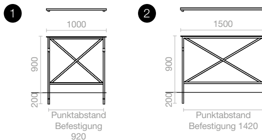
Befestigungsprinzip
