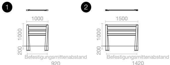
Befestigungsprinzip
