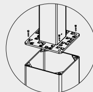
Befestigungsprinzip
