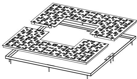
Befestigungsprinzip
