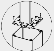
Befestigungsprinzip mit Punktabstand
