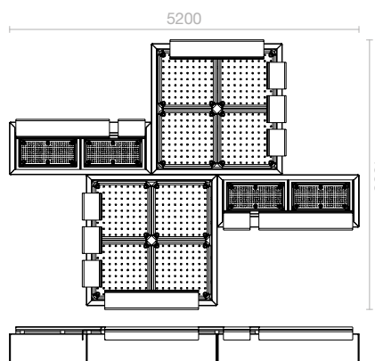
(D) 1-2-2-1
