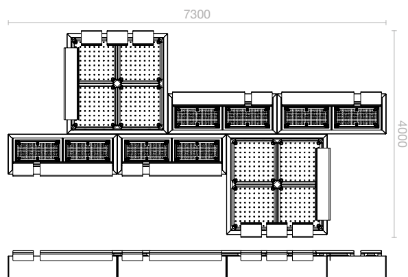
(E) 2-1-1-1-1-2
