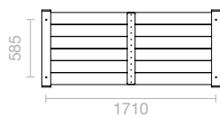
Vue de dessous (avec entraxes de fixation)
