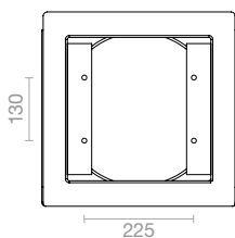
Vue de dessous (avec entraxes de fixation)
