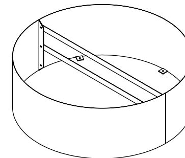
Durchmesser Ø140 mm bzw. Ø1800 mm, zweiteilig
