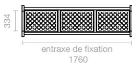
Vue de dessous (avec entraxes de fixation)
