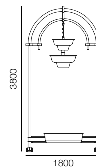
ARCEAU CAMÉLIA CAMELIA ARCH
