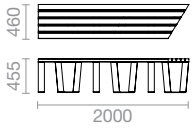
Befestigungsprinzip
