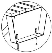
Befestigungsprinzip
